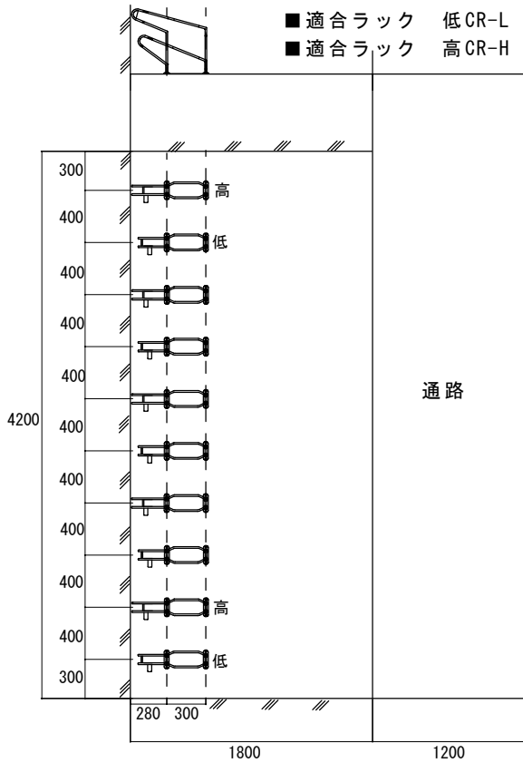
① 高低配列片側直角置
