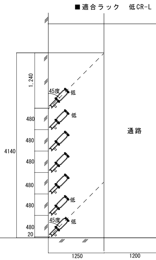
② 低配列斜角45度置
