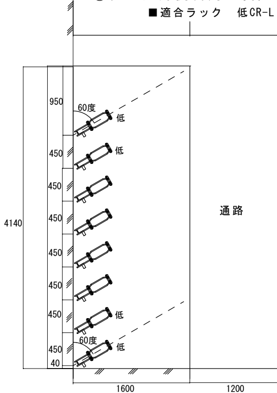
③ 低配列片側斜角60度置
